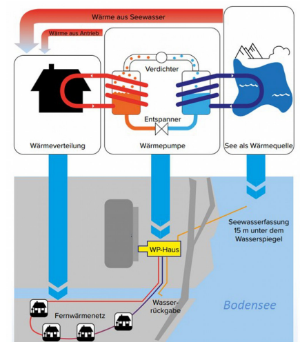
Schema Seewasserwärmenutzung
