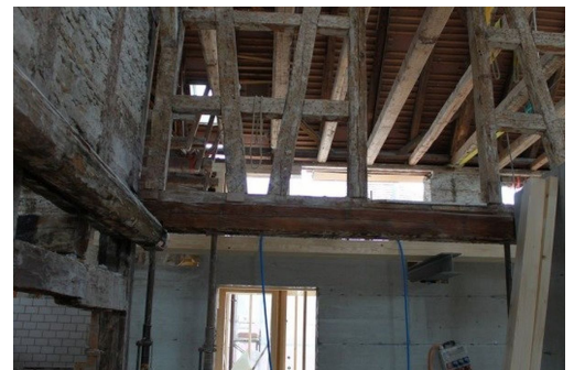
Bestehende Holzkonstruktion
