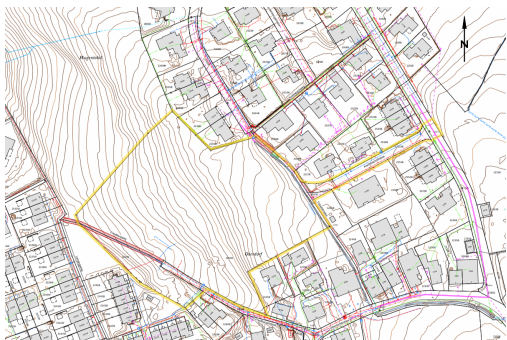
Situation Planungsbereich
